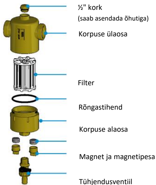
Joonis 3: FAR õhuseparaator – ehitus
