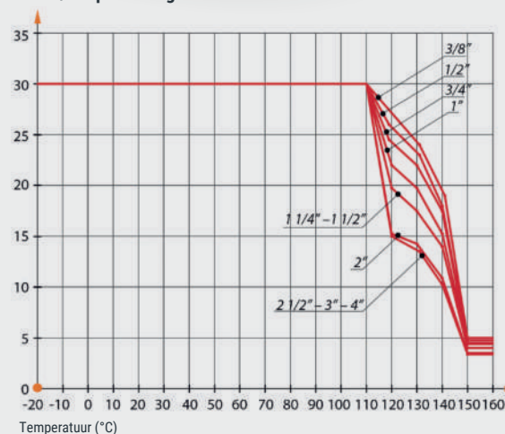
Rõhu-/temperatuurigraafik
