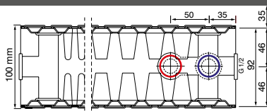
tüüp 22 plus / tüüp 22 sügavus 100 mm
