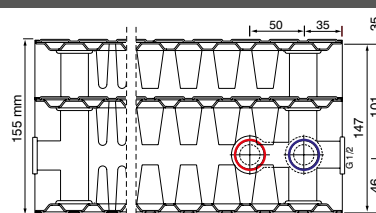
tüüp 33 plus / tüüp 33 sügavus 155 mm
