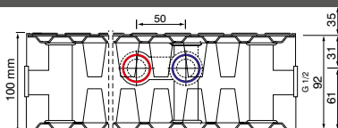
tüüp 22 sügavus 100 mm
