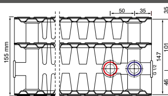
tüüp 33 plus / tüüp 33 sügavus 155 mm pr
