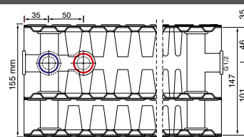
tüüp 33 / tüüp 33 plus sügavus 155 mm pl
