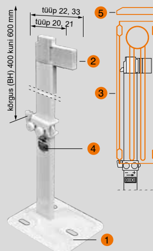
põrandakandur „Standard“ kõrgused 400–600
