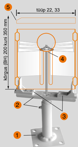
põrandakandur „Plus“ kõrgused 200/350
