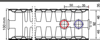
tüüp 22 plus / tüüp 22 sügavus 100 mm pr
