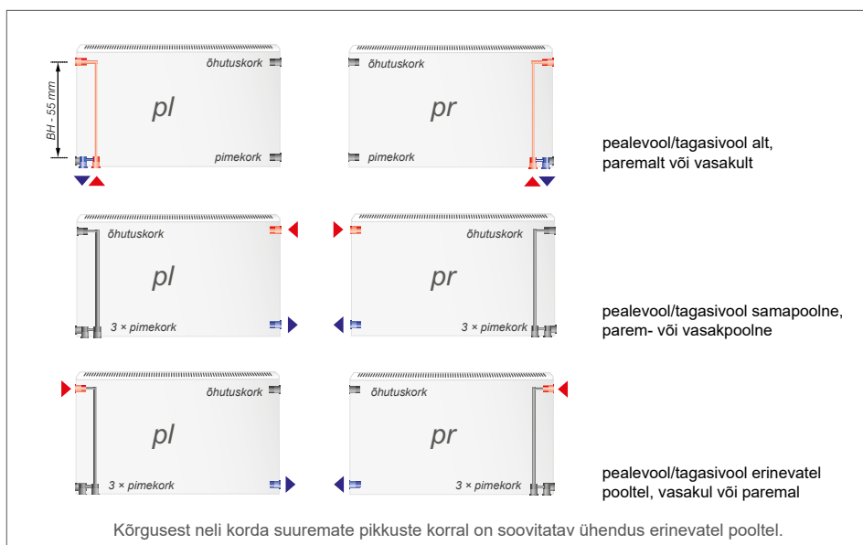
tüüp 33 sügavus 155 mm pr
