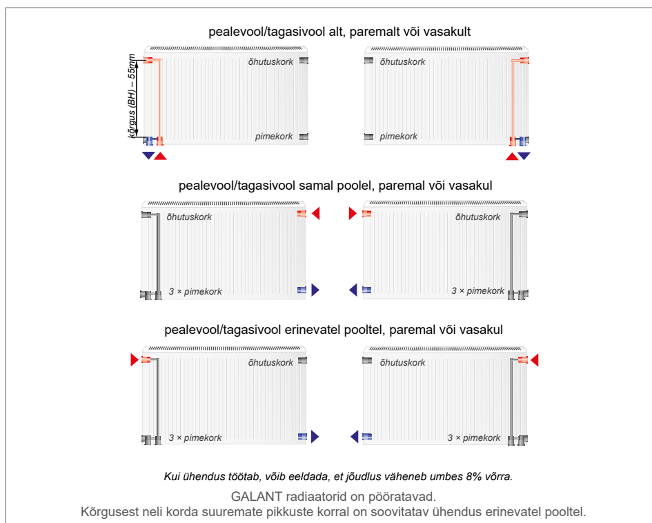
tüüp 22 plus / tüüp 22 sügavus 100 mm
