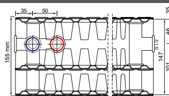
tüüp 33 sügavus 155 mm pl
