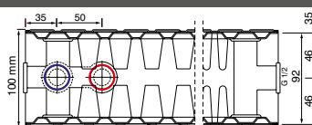
tüüp 22 / tüüp 22 plus sügavus 100 mm pl
