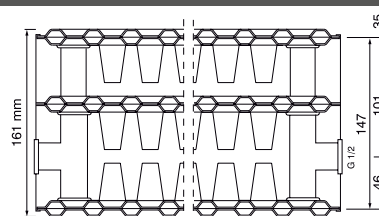
tüüp 33 sügavus 161 mm
