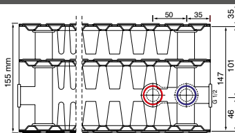
tüüp 33 sügavus 155 mm pr
