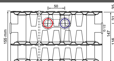
tüüp 33 sügavus 155 mm
