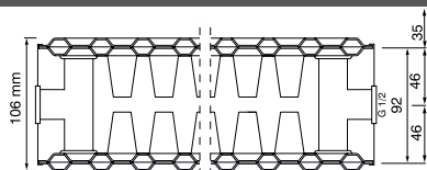
tüüp 22 sügavus 106 mm
